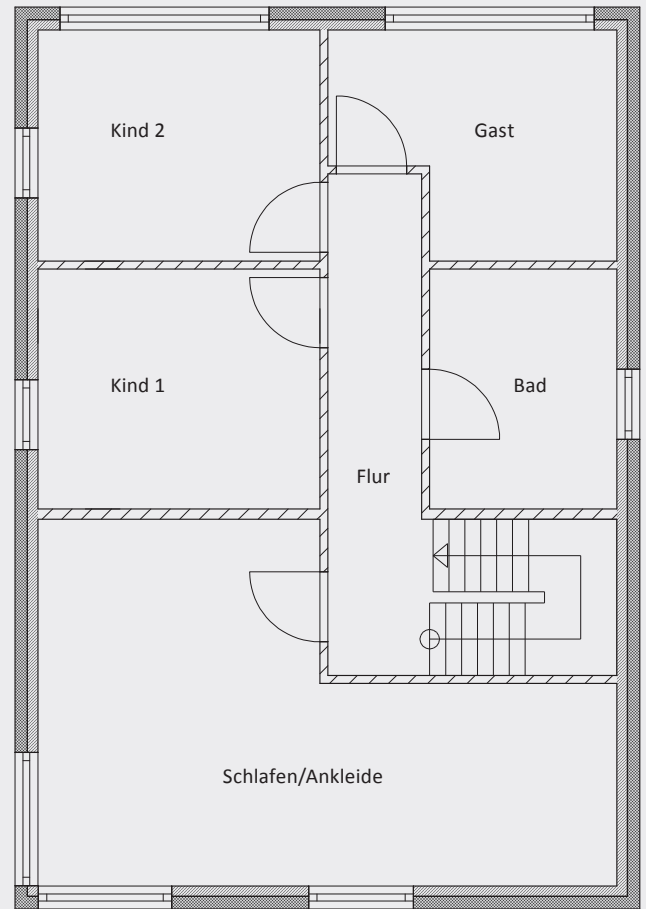
Grundriss Obergeschoss
