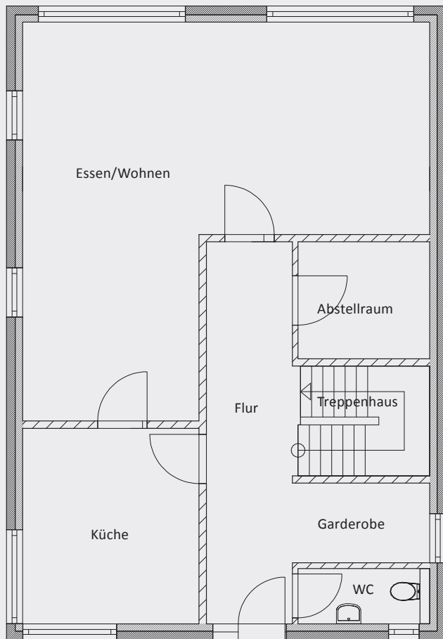
Grundriss Erdgeschoss
